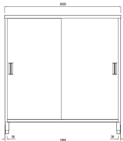
Fronte
