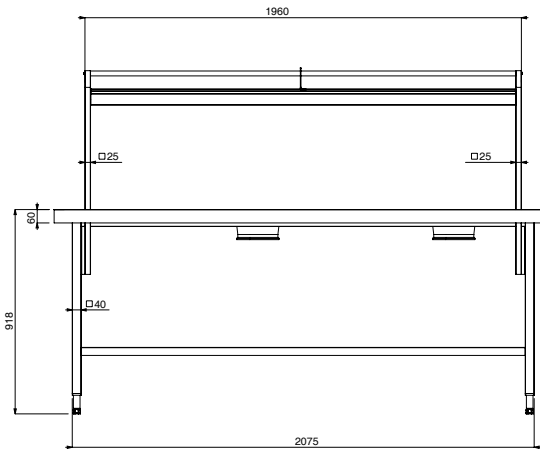
Alzado
